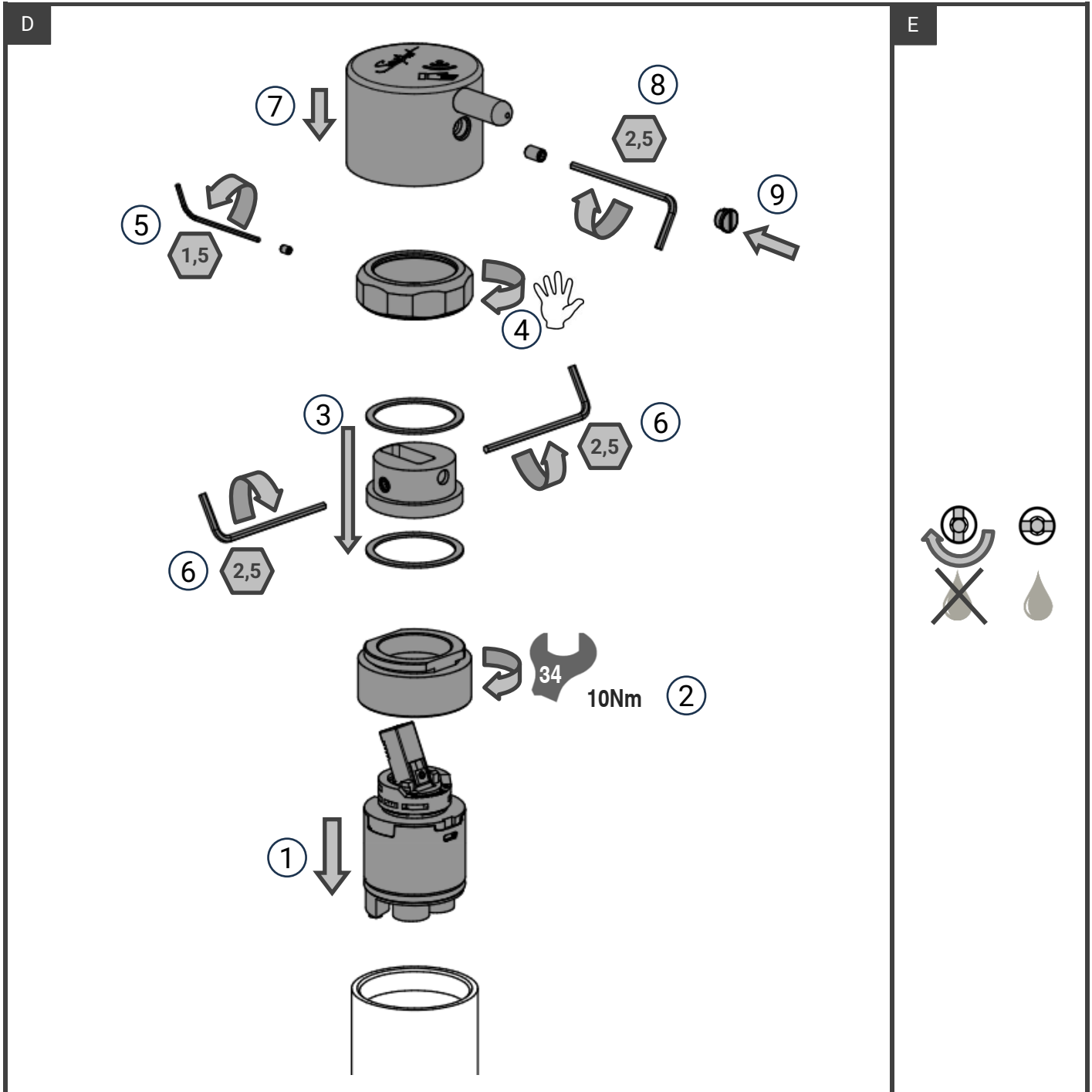
5-2 Maintenance Bec Démontable/ Maintenance of removable spout/ Wartung abnehmbarer Auslauf/ Mantenimiento del caño desmontable/ Manutenzione della bocca smontabile/ Onderhoud van demonteerbare uitloop
