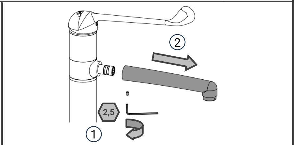
5-2 Maintenance Bec Démontable/ Maintenance of removable spout/ Wartung abnehmbarer Auslauf/ Mantenimiento del caño desmontable/ Manutenzione della bocca smontabile/ Onderhoud van demonteerbare uitloop
